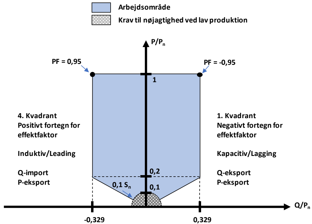
Figur 4.8 – Krav til levering af reaktiv effekt ved forskellige niveauer af aktiv effekt.
