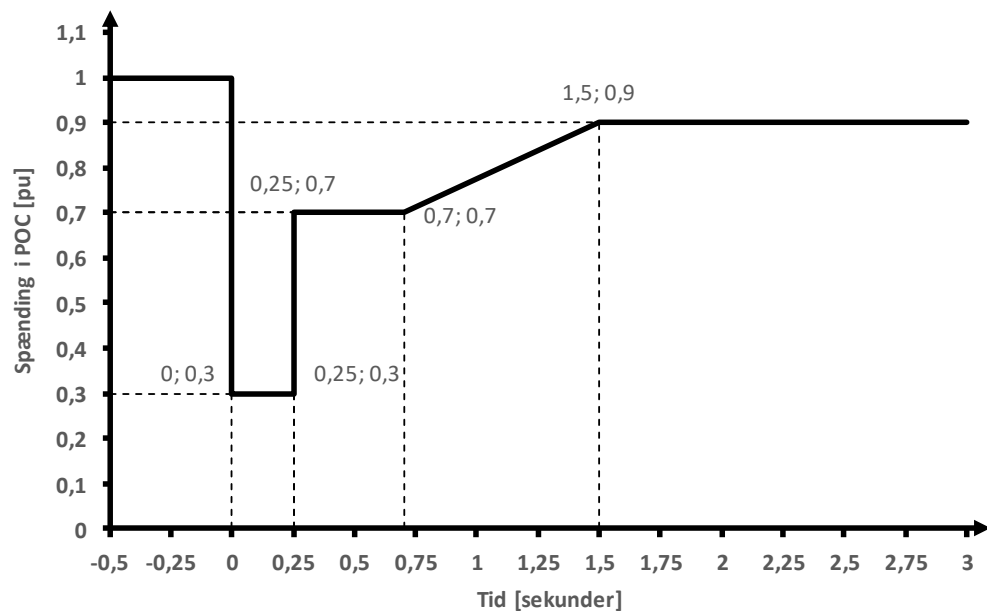
Figur 4.3 – Robusthed over for spændingsdyk for et synkront produktionsanlæg.
