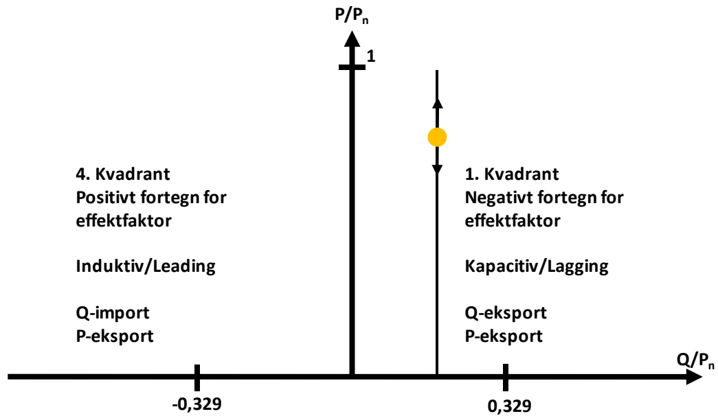
Figur 5.15 – Eksempel på Q-regulering [Q setpunkt].
