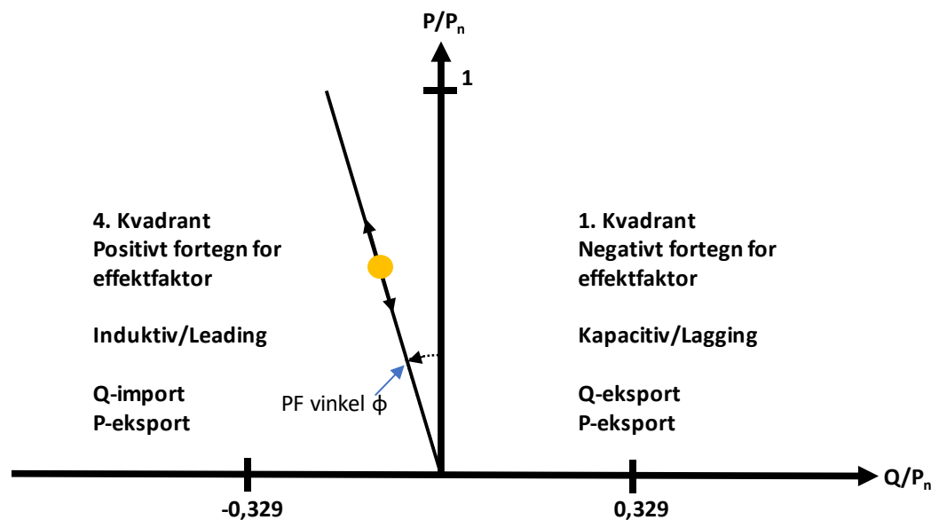
Figur 6.13 – Eksempel på effektfaktorregulering [ \cos \phi fix].
